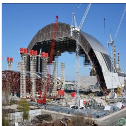
Sarcofagul de beton în construcție deasupra reactorului nr. 4 avariat (etapa de construcție și montaj)
