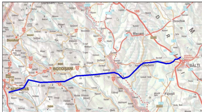
Traseu LEA 400 kV SUCEAVA (România) - BĂLȚI (Moldova)
